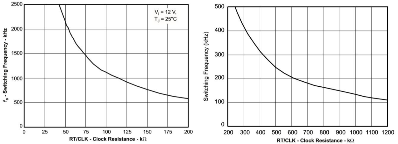
图 9 频率与 RT 下拉电阻的关系
