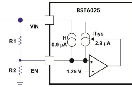
图 7 可调整的 uvlo 电压
