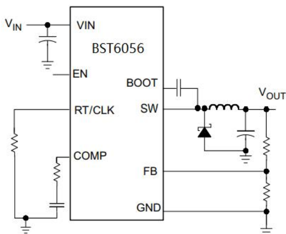
图 2 BST6056 简化应用电路
