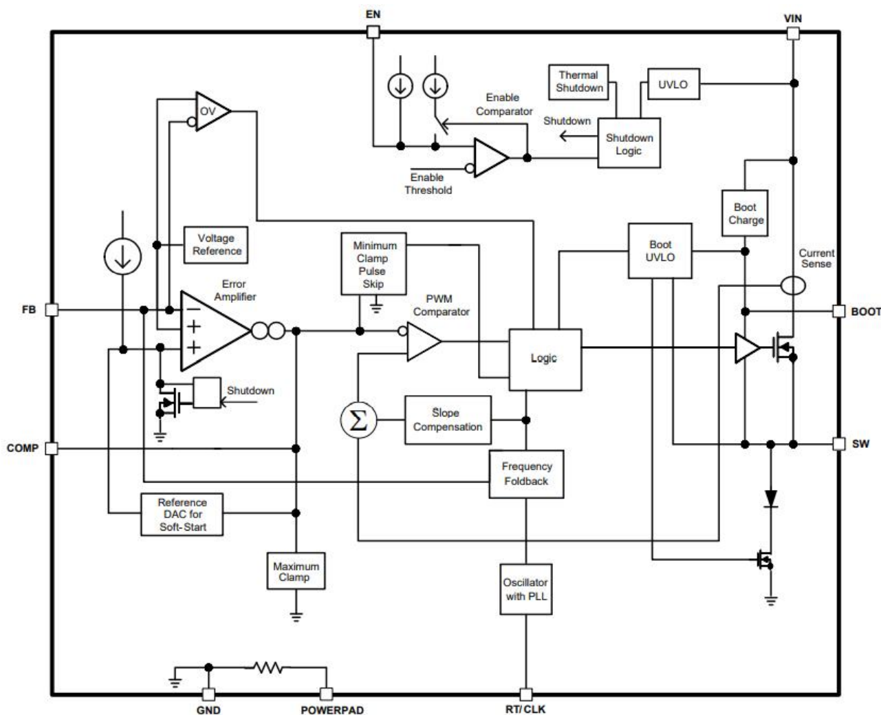
图 1 BST6056 内部模块框图
