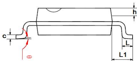
端视图
