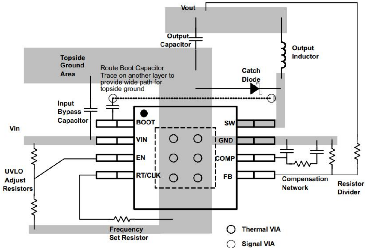
图 11 PCB layout 参考示意图
