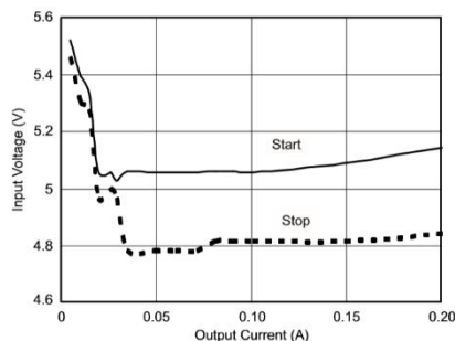
图 4 5V 启动和关闭电压
