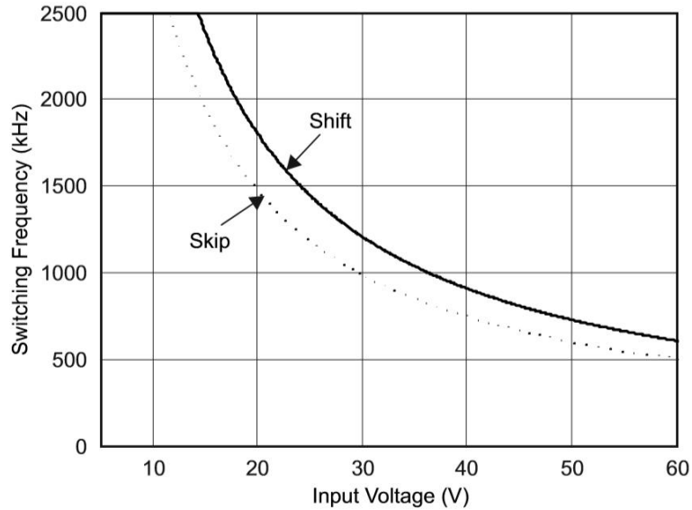
图 10 最大开关频率与输入电压的关系
