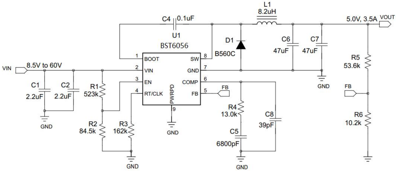
图 3 输出 5V 典型应用线路
