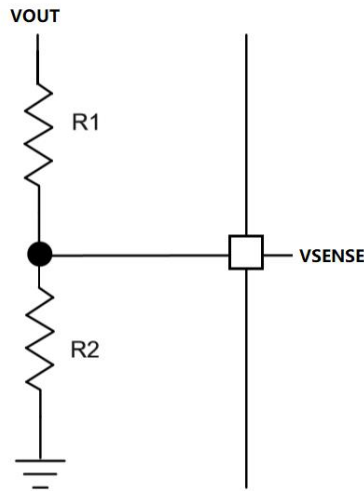
图 6 通过 VSENSE 设置输出电压
