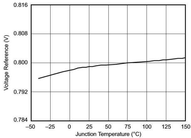
图 5 基准电压的温度特性
