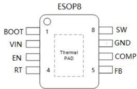
图 1 引脚示意图
