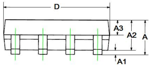
侧视图
