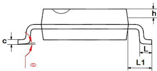
端视图
