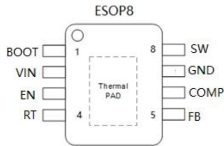
图 1 引脚示意图
