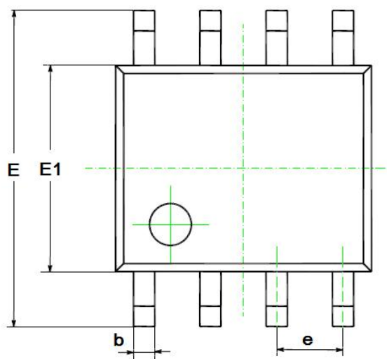
顶视图
