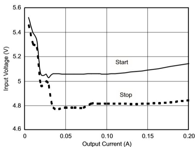
图 4 5V 启动和关闭电压
