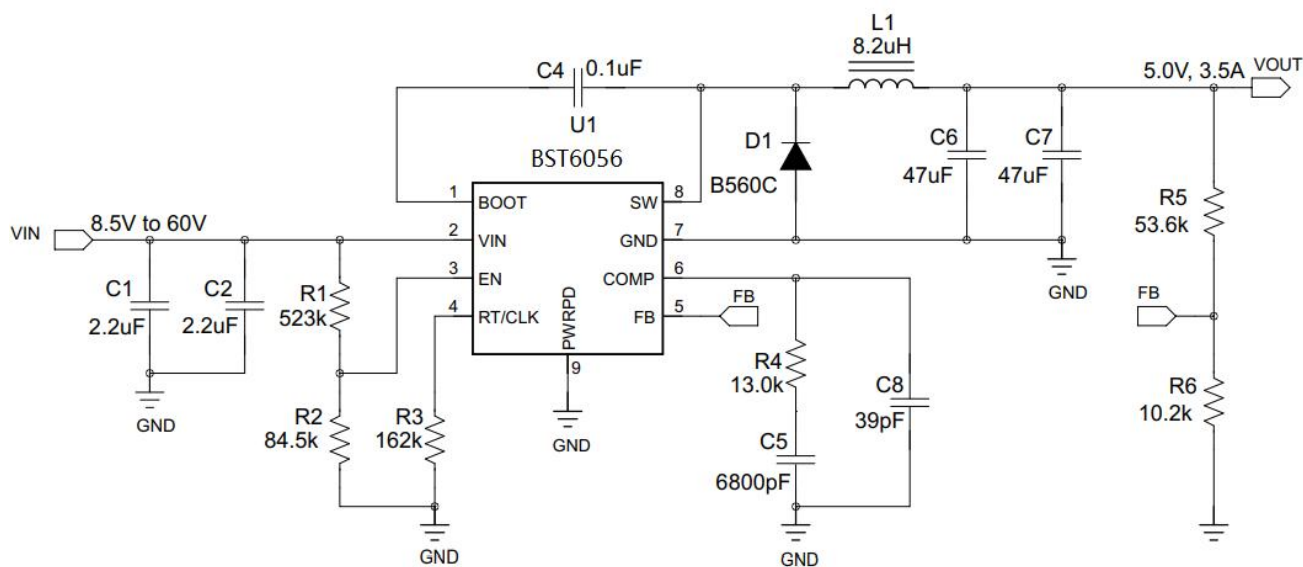
图 3 输出 5V 典型应用电路
