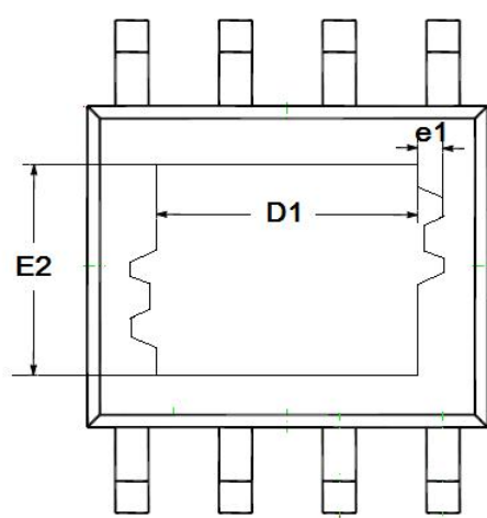
底视图
