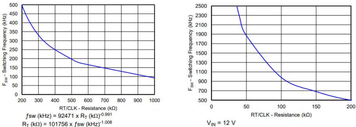
图 11 频率与 RT 下拉电阻的关系
