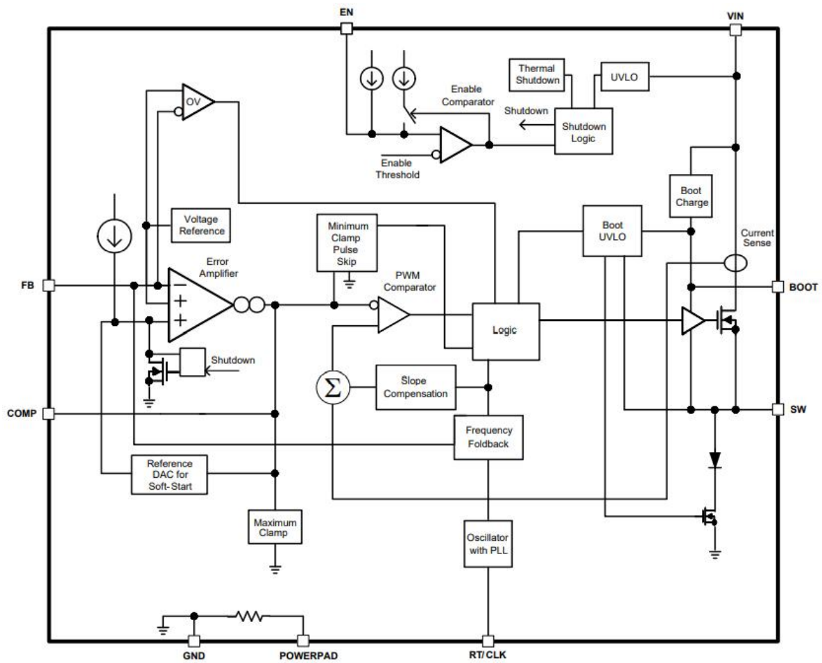
图 1 BST6056 内部模块框图
