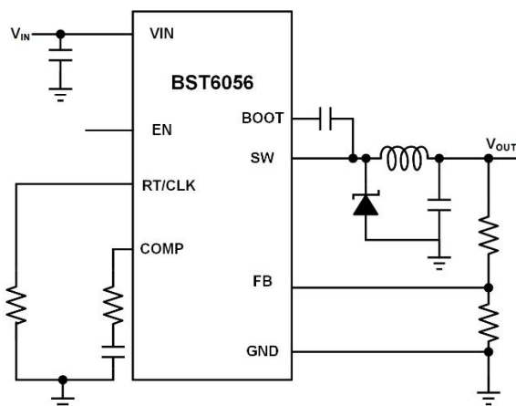
图 2 BST6056 简化应用电路
