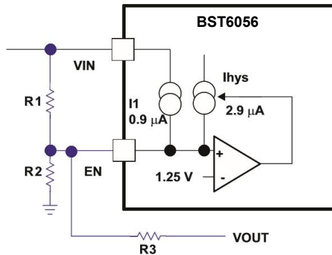
图 8 增加额外的滞回系数
