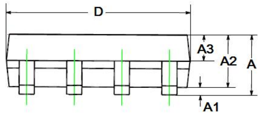
侧视图
