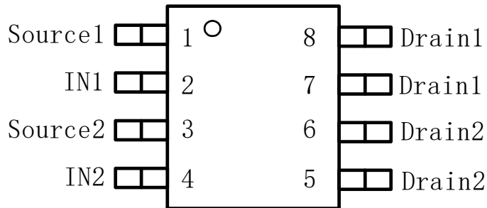
图4-1 SOP8管脚排列图
