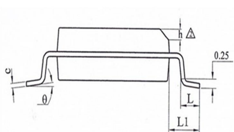
图8-2 MCS4235S封装规格SOT23-3L
