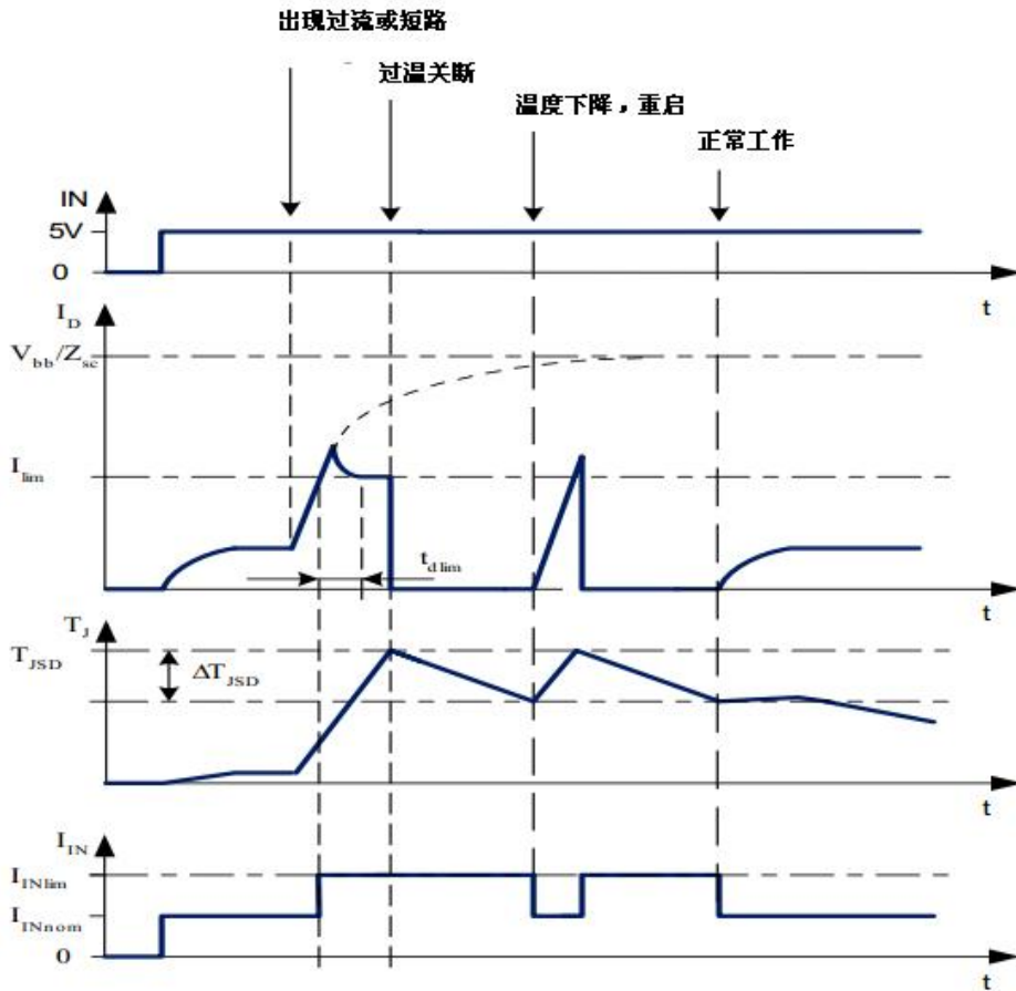
图7-2 MCS4235短路特性
