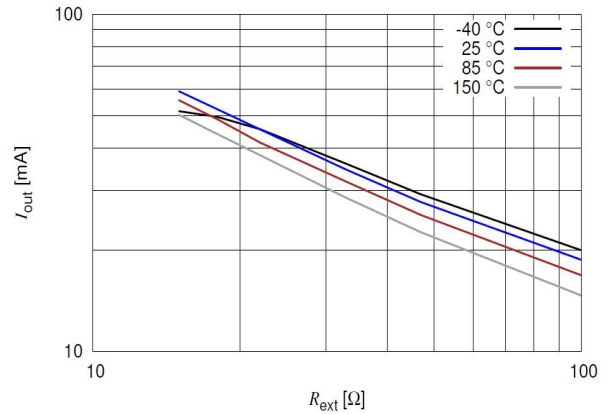
输出电流与外接电阻
