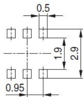
图 7 焊盘尺寸
