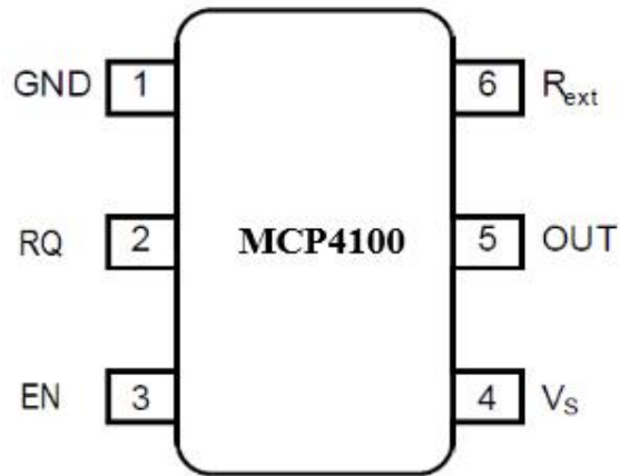
图 2 MCP4100C (SOT23-6)的引脚定义图
