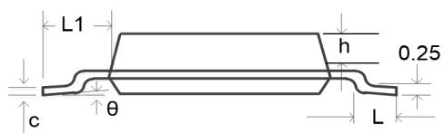
图8 SSOP10L封装尺寸
