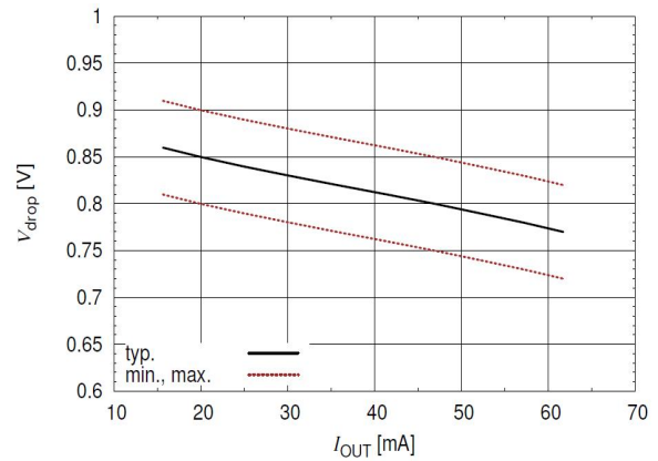
压降与输出电流
