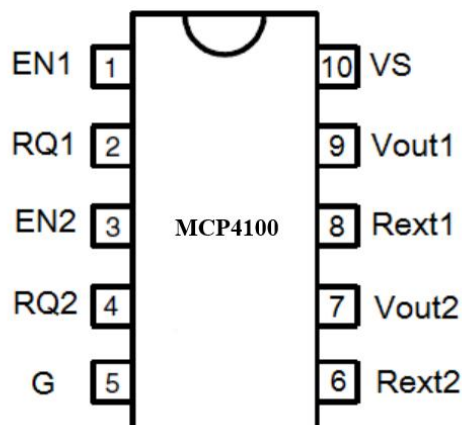
图 3 MCP4100C2 (SSOP10L)的引脚定义图
