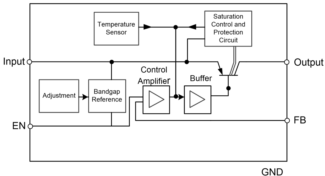
图 3 BST6008LADJ 内部模块框图（示意图）
