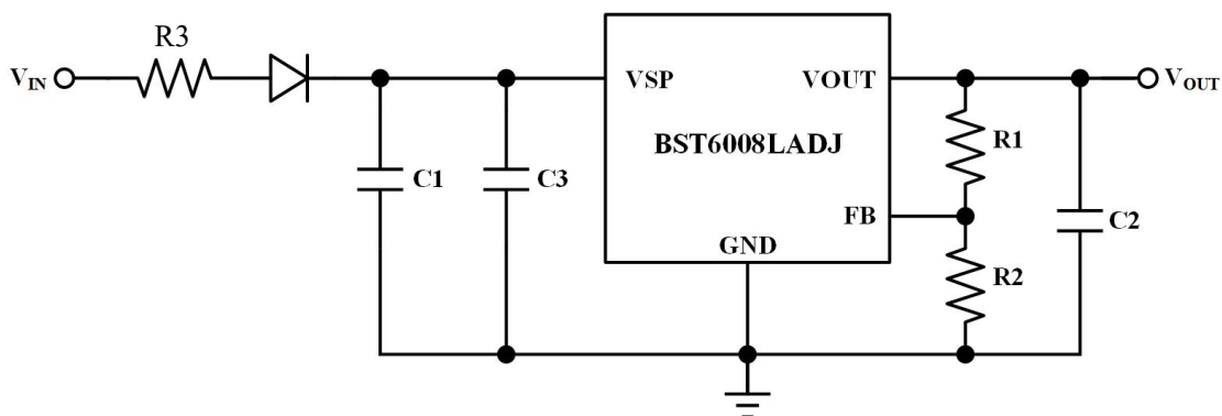
图 1 BST6008LADJ 典型应用电路
