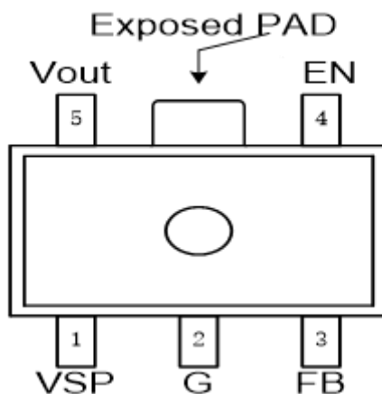
图 2 引脚定义图
