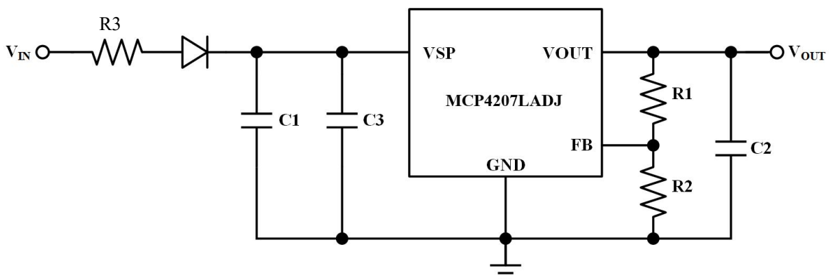
图 1 MCP4207LADJ 典型应用电路
