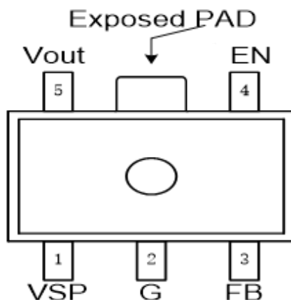
图 2 引脚定义图
