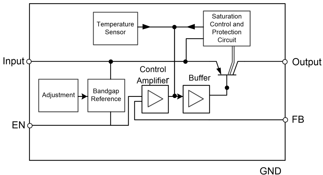
图 3 MCP4207LADJ 内部模块框图（示意图）
