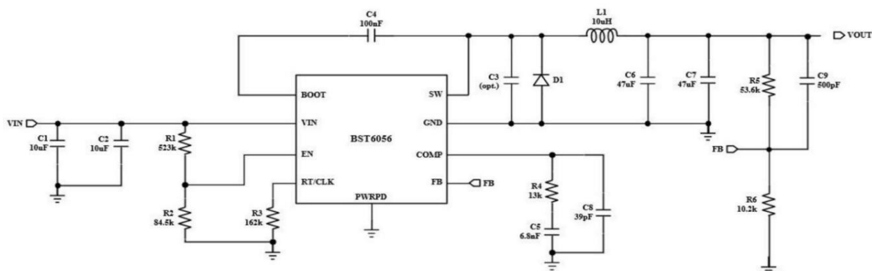
图 1 典型应用电路（输出电压5V）
