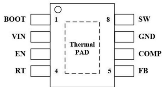
图 2 引脚定义图
