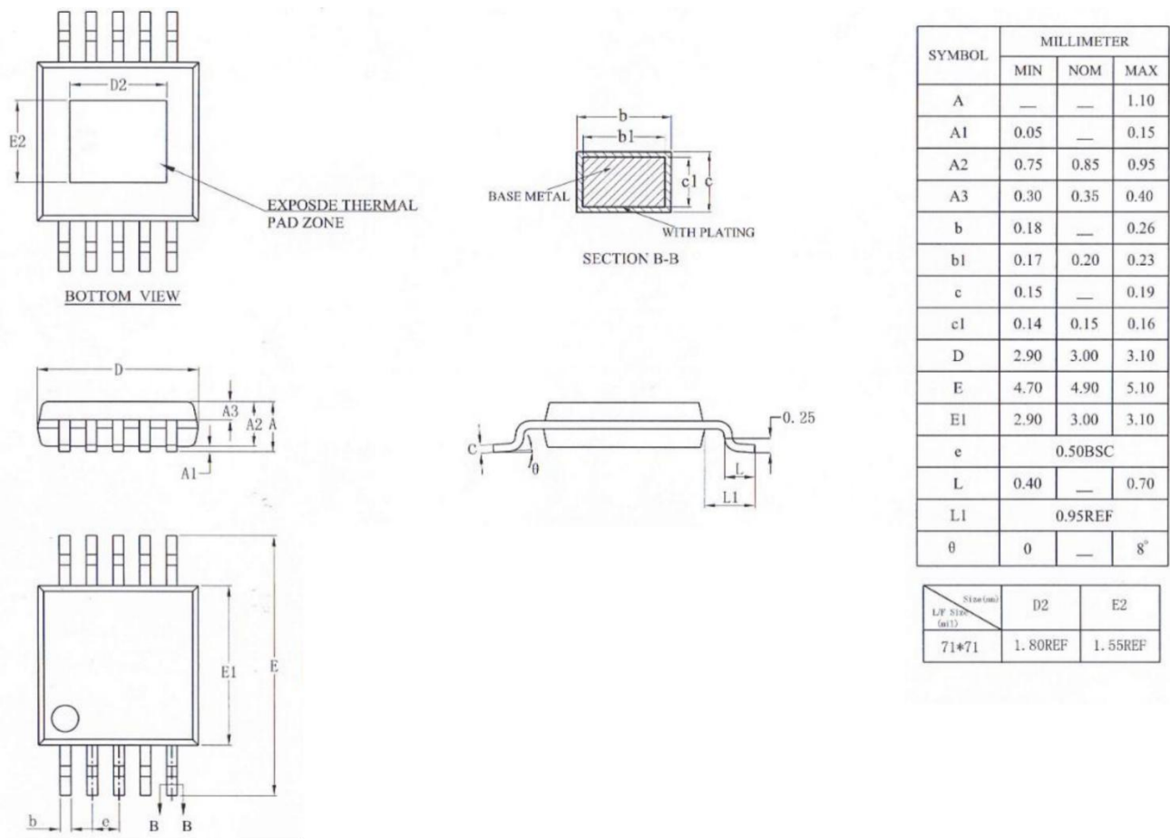
EMSOP10 封装外形图
