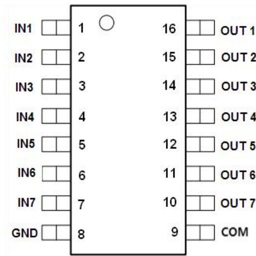
图 3 引脚定义图
