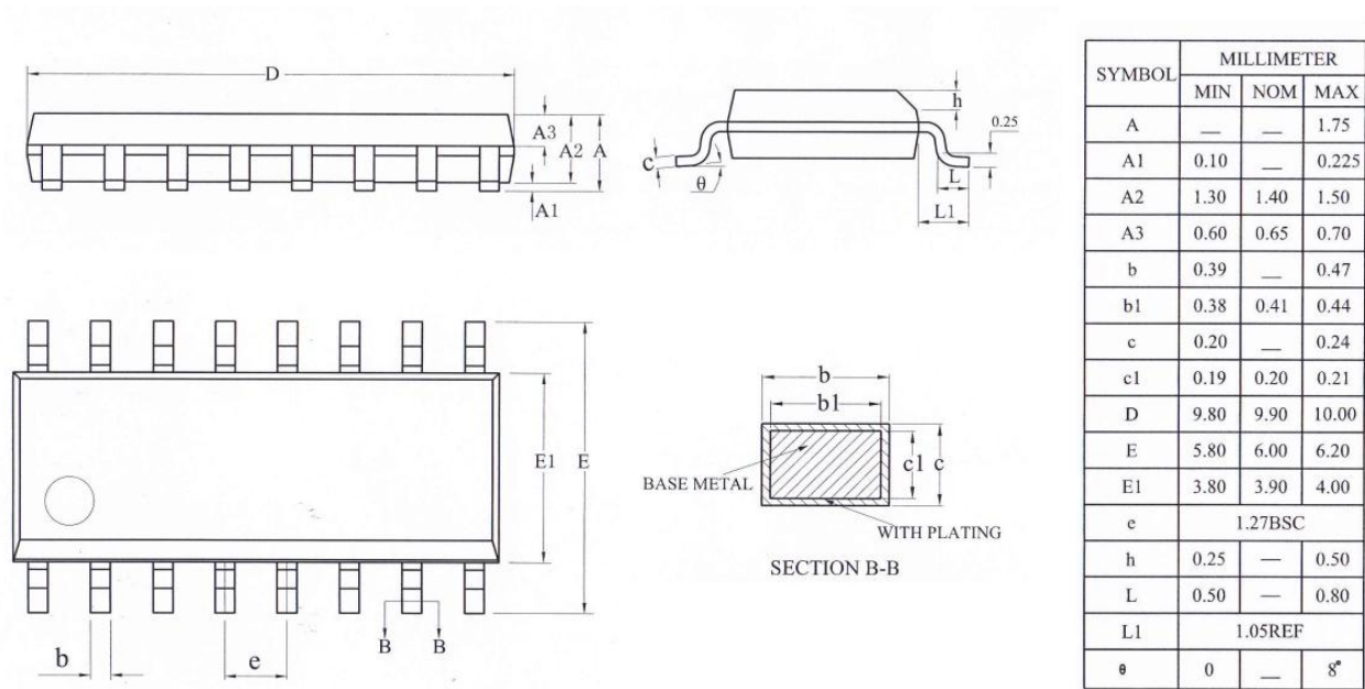
SOP16L 封装外形图
