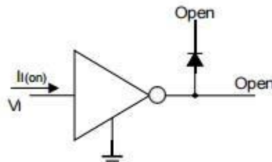
图 4 II(on)测试电路图
