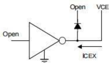
图 1 ICEX测试电路图
